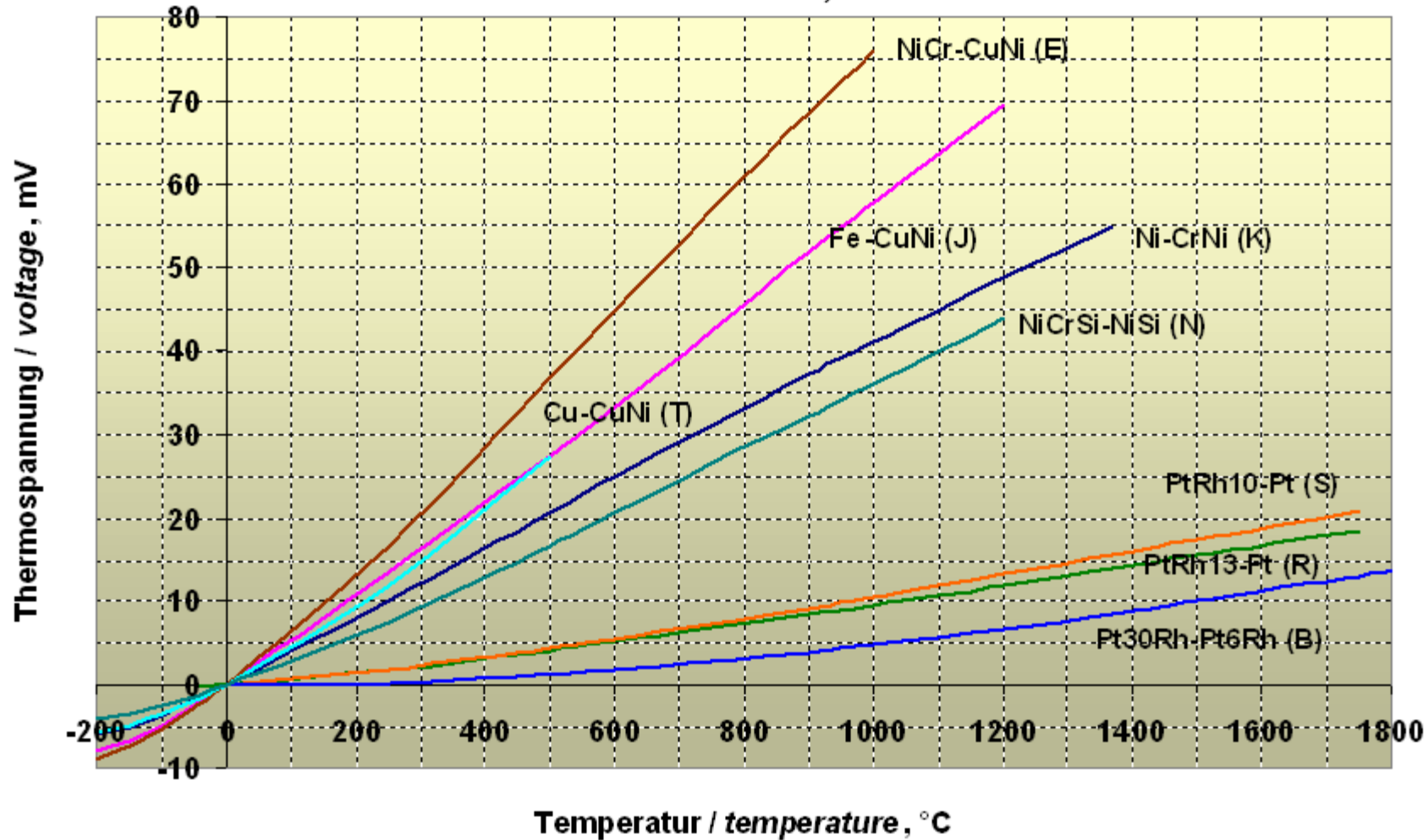
Thermospannungen verschiedener Thermopaare bezogen auf eine Vergleichsstellentemperatur von 0°C (DIN EN 60 584) Voltages of different thermocouples relativ to a reference temperature of 0°C (according to DIN EN 60584)
